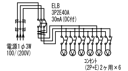
結線図
